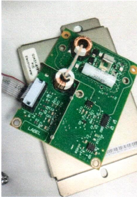
Part bagian Electrometer Bagian dalam
