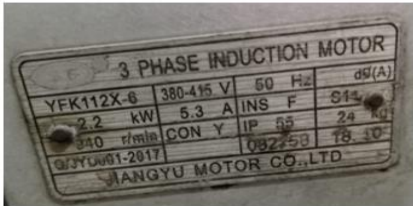
Name Plate motor fan chiller
